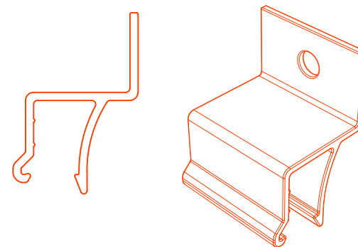
FP PLANK CLIP
