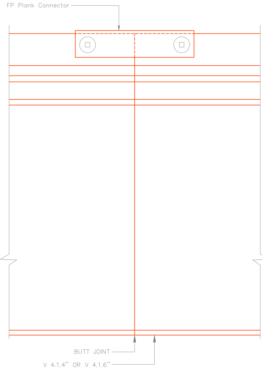
ELEVATION
